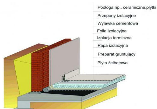
Podłoga na gruncie w budynku podpiwniczonym
